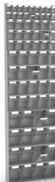
SCAFFALE CON 72 CASSETTI VISUAL BOX DIM. (mm): L=602 P=190 H=2000
