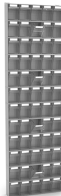
SCAFFALE CON 60 CASSETTI VISUAL BOX DIM. (mm): L=602 P=157 H=2000
